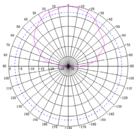
Horizontal Pattern 698-960 & 1710-2700MHz
